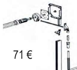
Acționare reductor cu manivelă pliabilă
