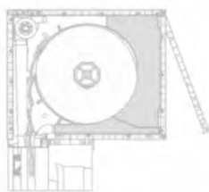
Capac vizitare partea exterioară, rulou suprapus
