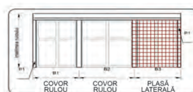
Rulouri cu casetă comună și plasă laterală
