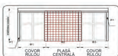
Rulouri cu casetă comună și plasă centrală
